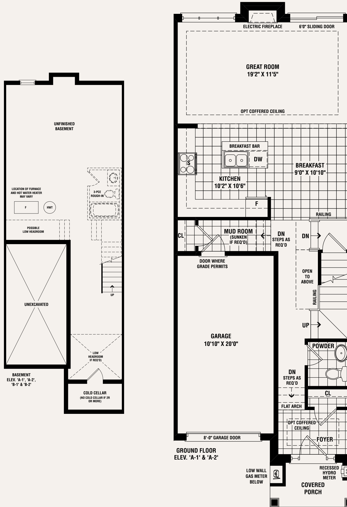
ELEVATION A
